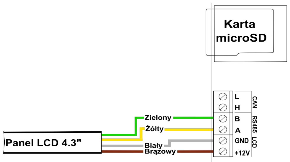
Ilustracja 2: Podłączenie panelu CD2/CD3 4.3" w sterowniku v4
