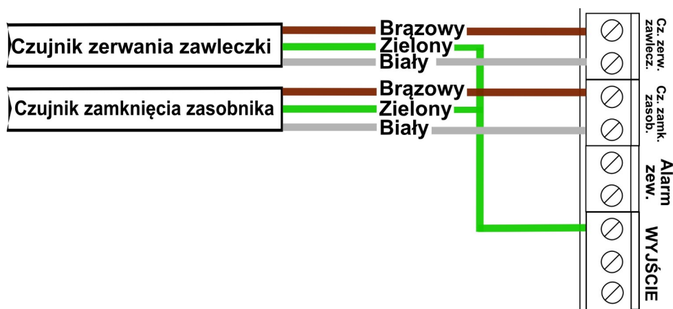
Ilustracja 3: Podłączenie czujników: zerwania zawleczki oraz zamknięcia zasobnika
