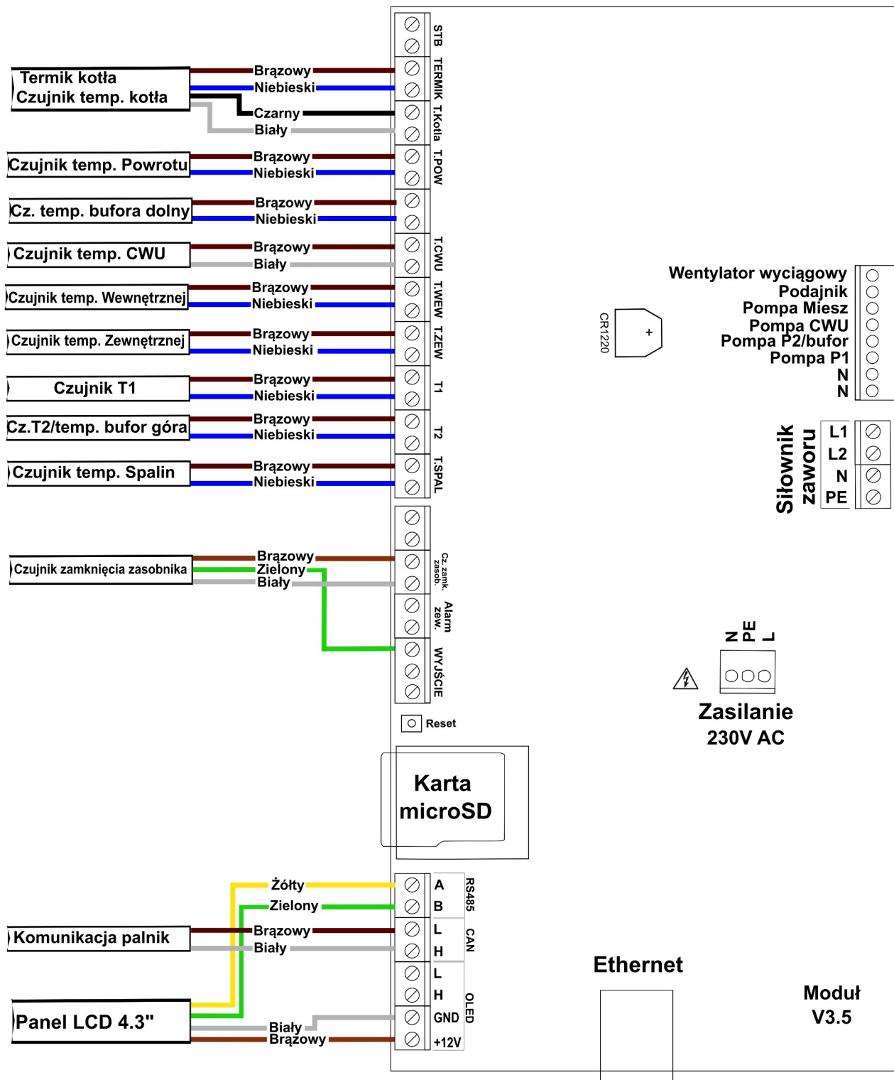
Ilustracja 7: Listwa zaciskowa do podłączenia sterownika v3.5
