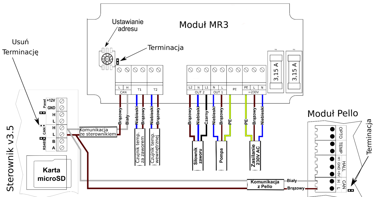
Ilustracja 12: Schemat podłączenia modułu rozszerzeń MR3 w sterowniku v3.5.
