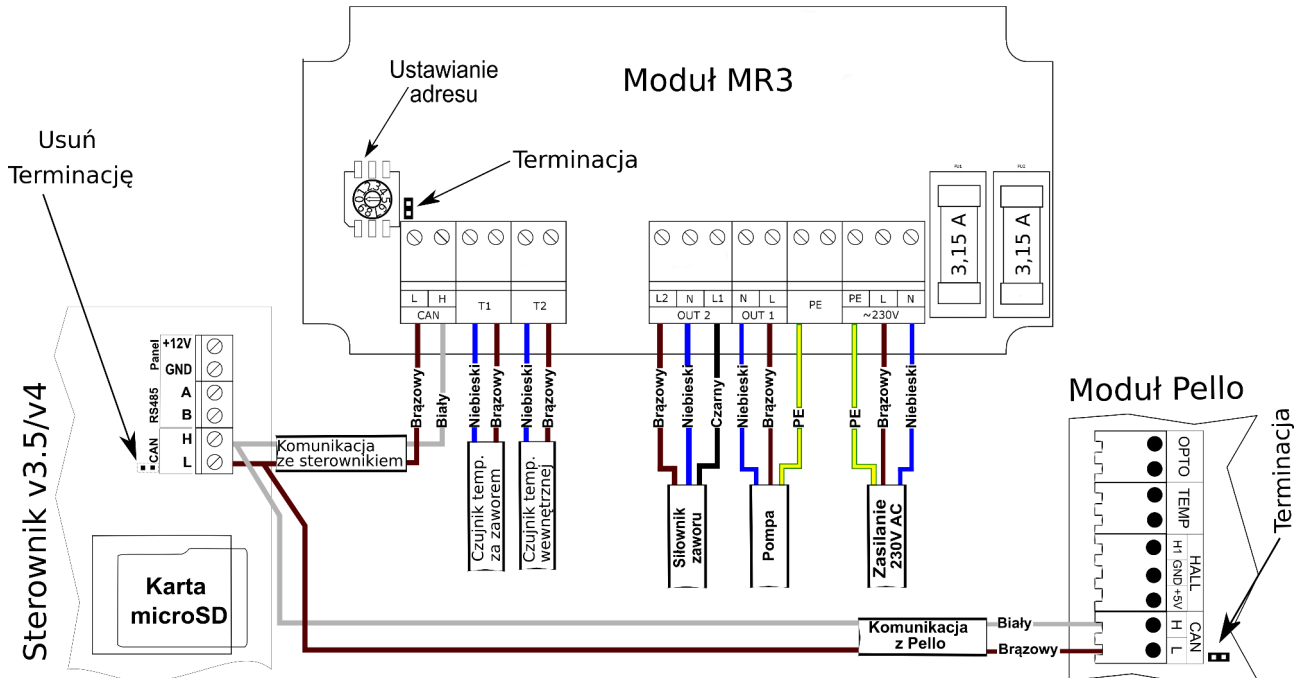
Ilustracja 11: Schemat podłączenia modułu rozszerzeń MR3 do sterownika v4.
