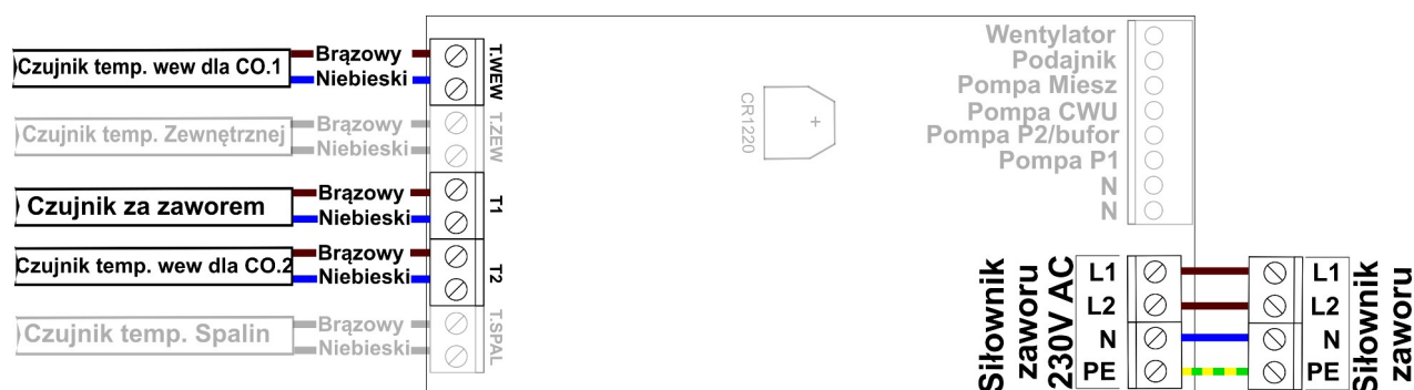
Ilustracja 8: Podłączenie siłownika zaworu oraz czujników wewnętrznych dla obwodu CO.1/CO.2
