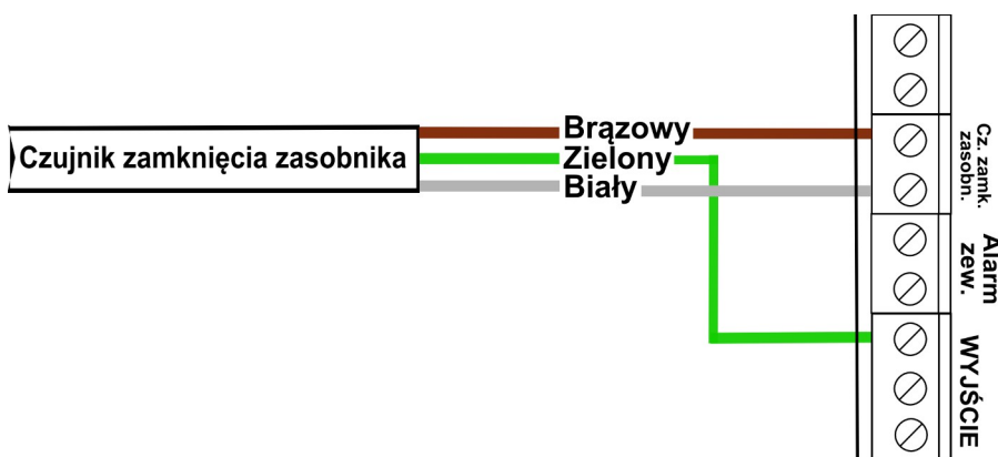
Ilustracja 10: Podłączenie czujnika zamknięcia zasobnika
