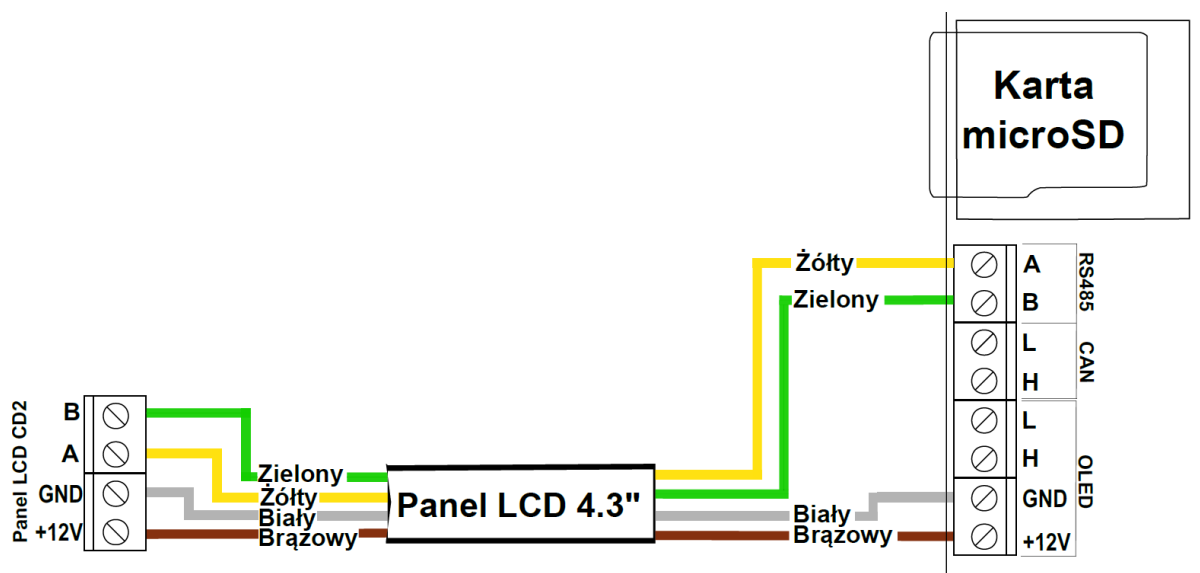
Ilustracja 2: Podłączenie przewodu panelu CD3/CD2 4.3" do sterownika v3.5
