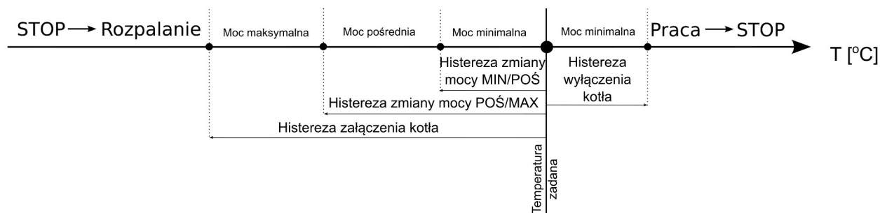
Ilustracja 24: Schemat przełączania się algorytmu spalania między mocami dla regulatora procesu spalania Auto
