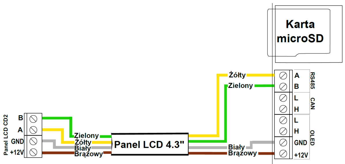
Ilustracja 2: Podłączenie panelu CD2 4.3" w sterowniku v3.5
