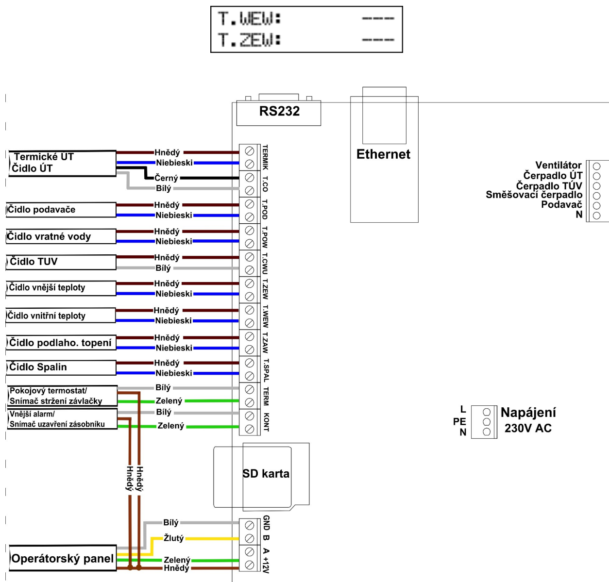
Ilustrace 3: Rozvodný pásek přípoje čidel
