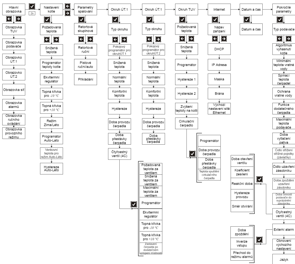
Obrázek 16: Schéma menu řídicí jednotky
