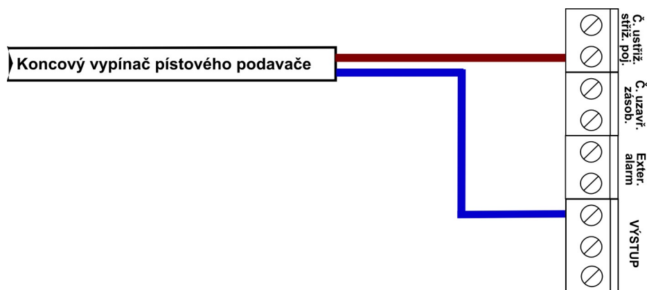
Obrázek 17: Zapojení koncového vypínače pístového podavače
