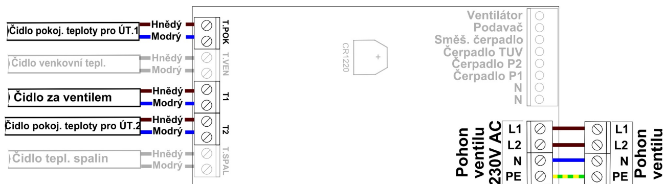
Obrázek 18: Zapojení pohonu ventilu a pokojových čidel pro okruh ÚT.1.
