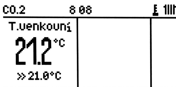
Obrázek 10: Obrazovka okruhu ÚT.2
