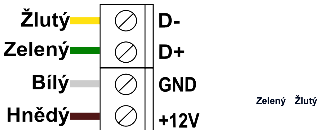
Obrázek 1: Zapojení panelu Standard
