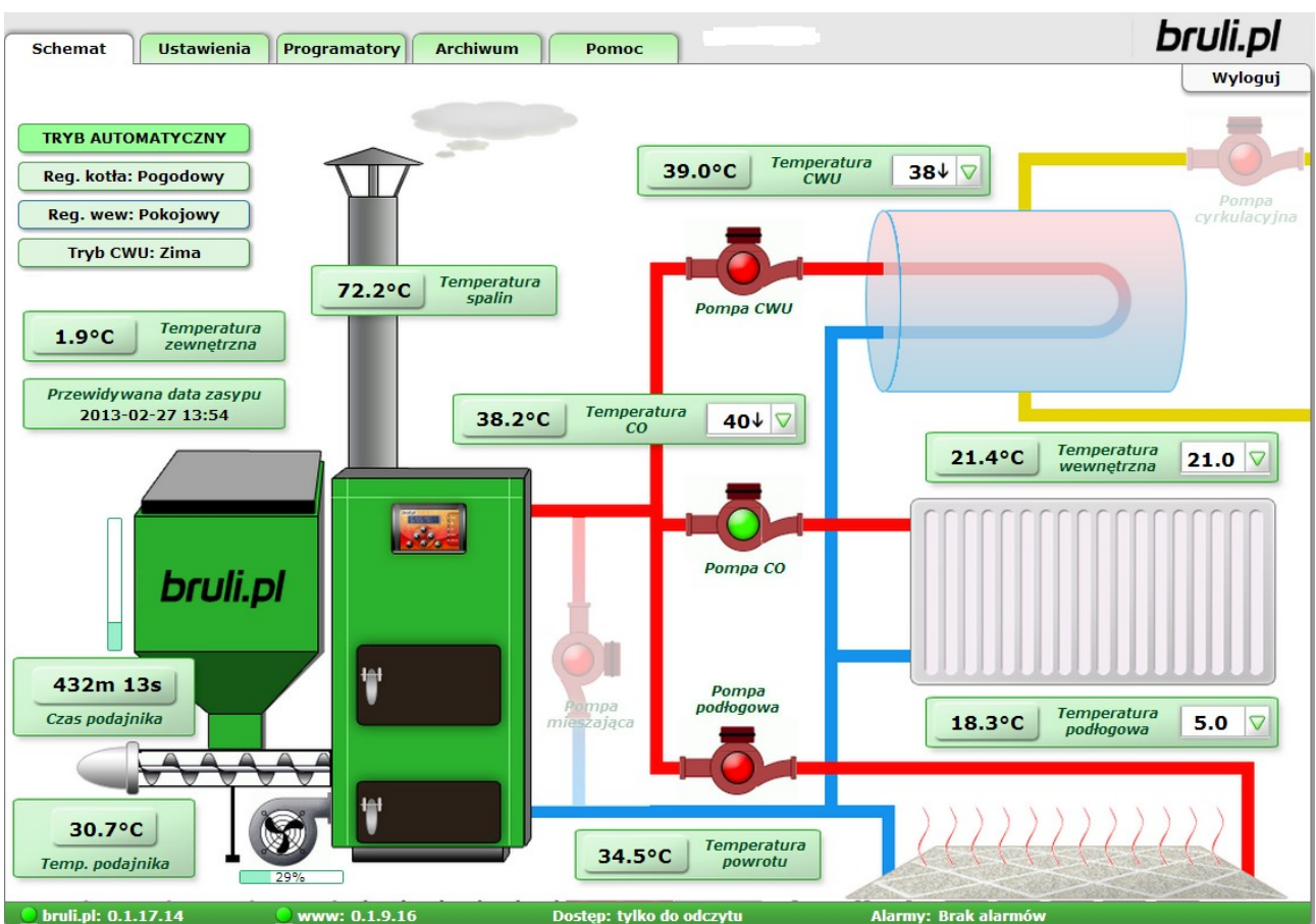
Ilustracja 18: Główne okno strony www w sterowniku bruli.pl
