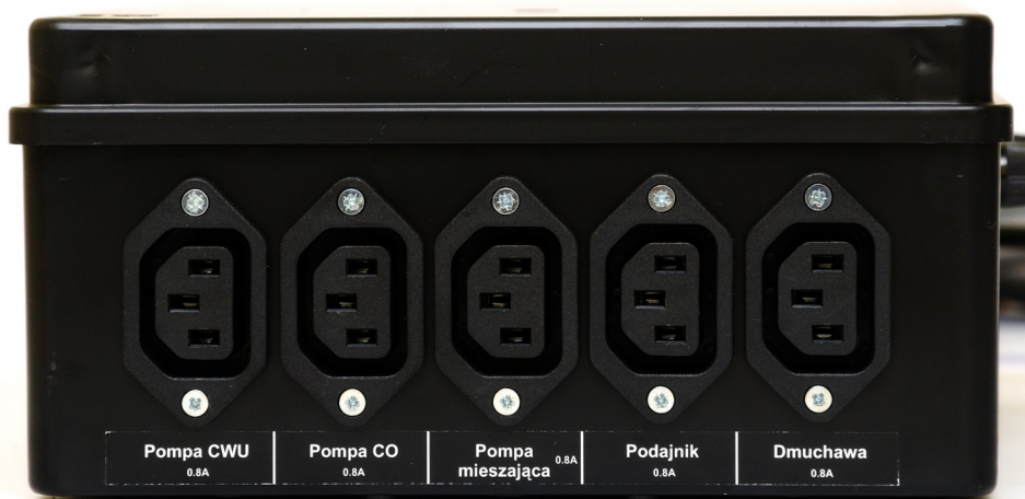
Ilustracja 5: Ścianka obudowy z wyjściami mocy
