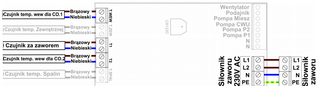
Ilustracja 17: Podłączenie siłownika zaworu oraz czujników wewnętrznych dla obwodu CO.1
