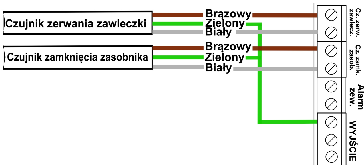
Ilustracja 3: Podłączenie czujników: zerwania zawlecarki oraz zamknięcia zasobnika
