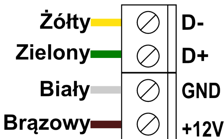
Ilustracja 1: Podłączenie panelu Standard
